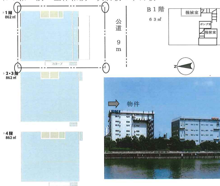
配置図兼1階平面図
